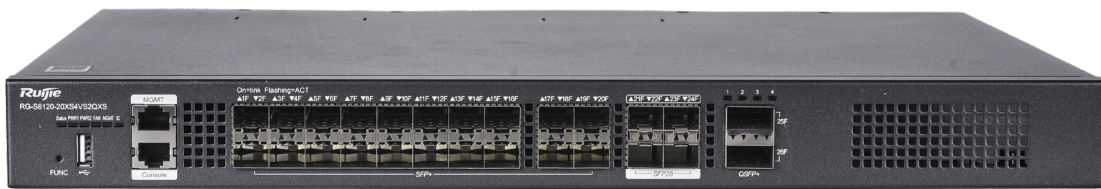
RG-S6120-20XS4VS2QXS正面俯视图
